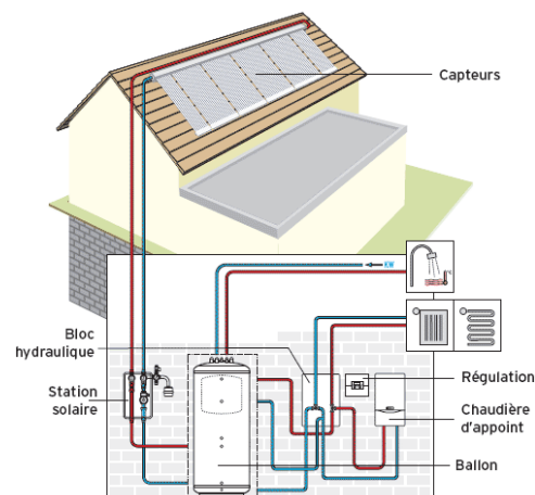
Figure 134 : Principe de fonctionnement d'une installation solaire thermique
